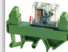
UDK2-RK 12Vdc 1NO
